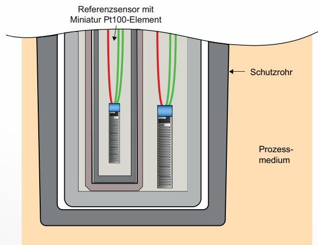
Abb. 3: Messeinsatz im Schutzrohr mit eingesetztem Referenzsensor
