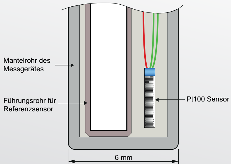
Abb. 2: Spitze eines Messeinsatzes mit zusätzlichen Kalibrierzugang
