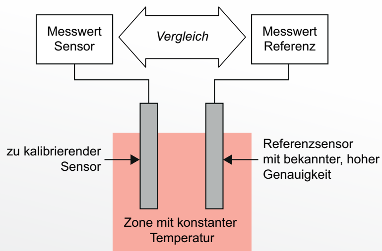
Abb. 1 Kalibrierprinzip für Temperaturmessgeräte
