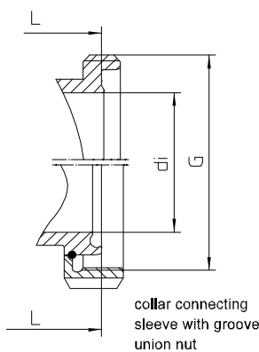
aseptic connection per DIN 11864-1
