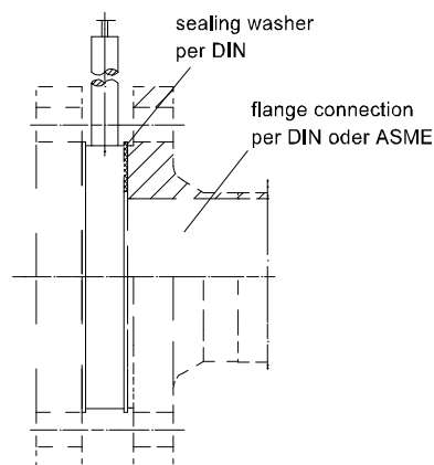
Dimensions (mm) per ASME B 16.5
